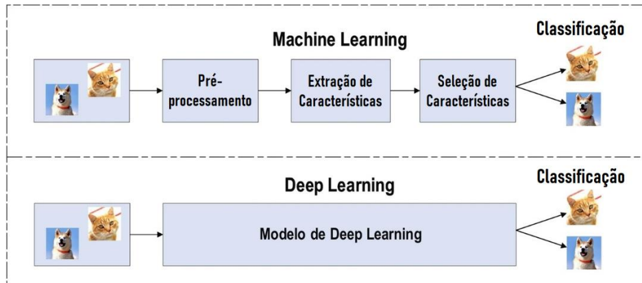
Figura 3 - Diferença entre deep learning e machine learning
