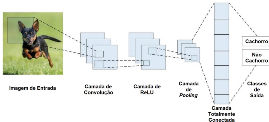
Figura 6 - Exemplo de uma arquitetura de redes neurais convolucionais para classificação de imagens
