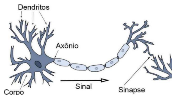
Figura 4 - Neurônio biológico
