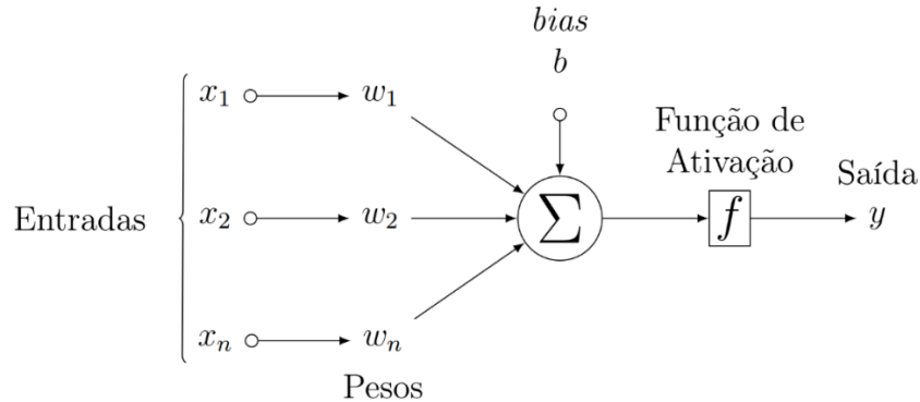
Figura 5 - Neurônio artificial
